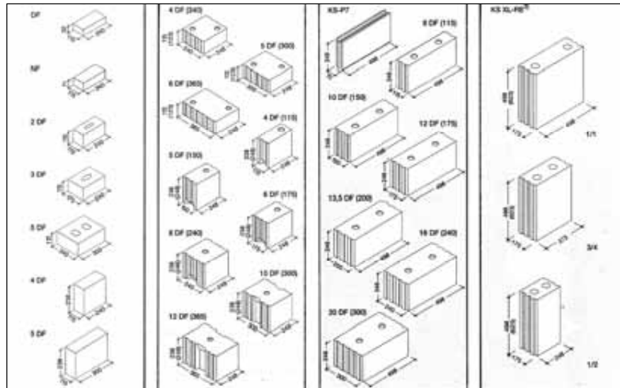
Kalksandstein-Formate und -Elemente.
